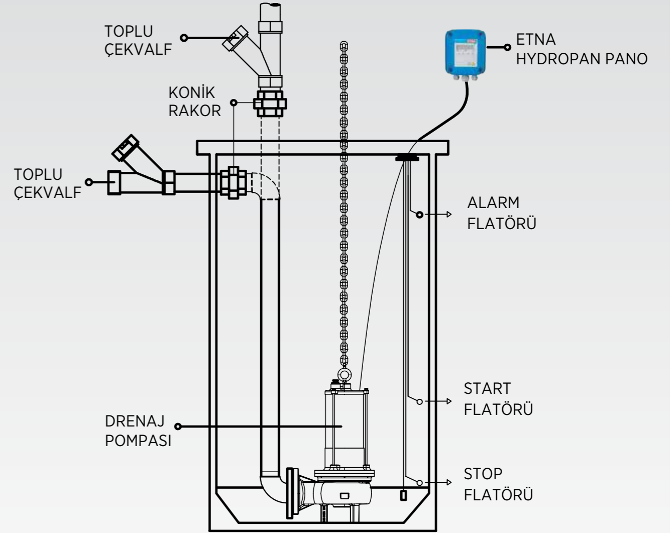
Sabit Tesisat (Bakım için Konik Rekordan Çıkarılabilir Pompa)
