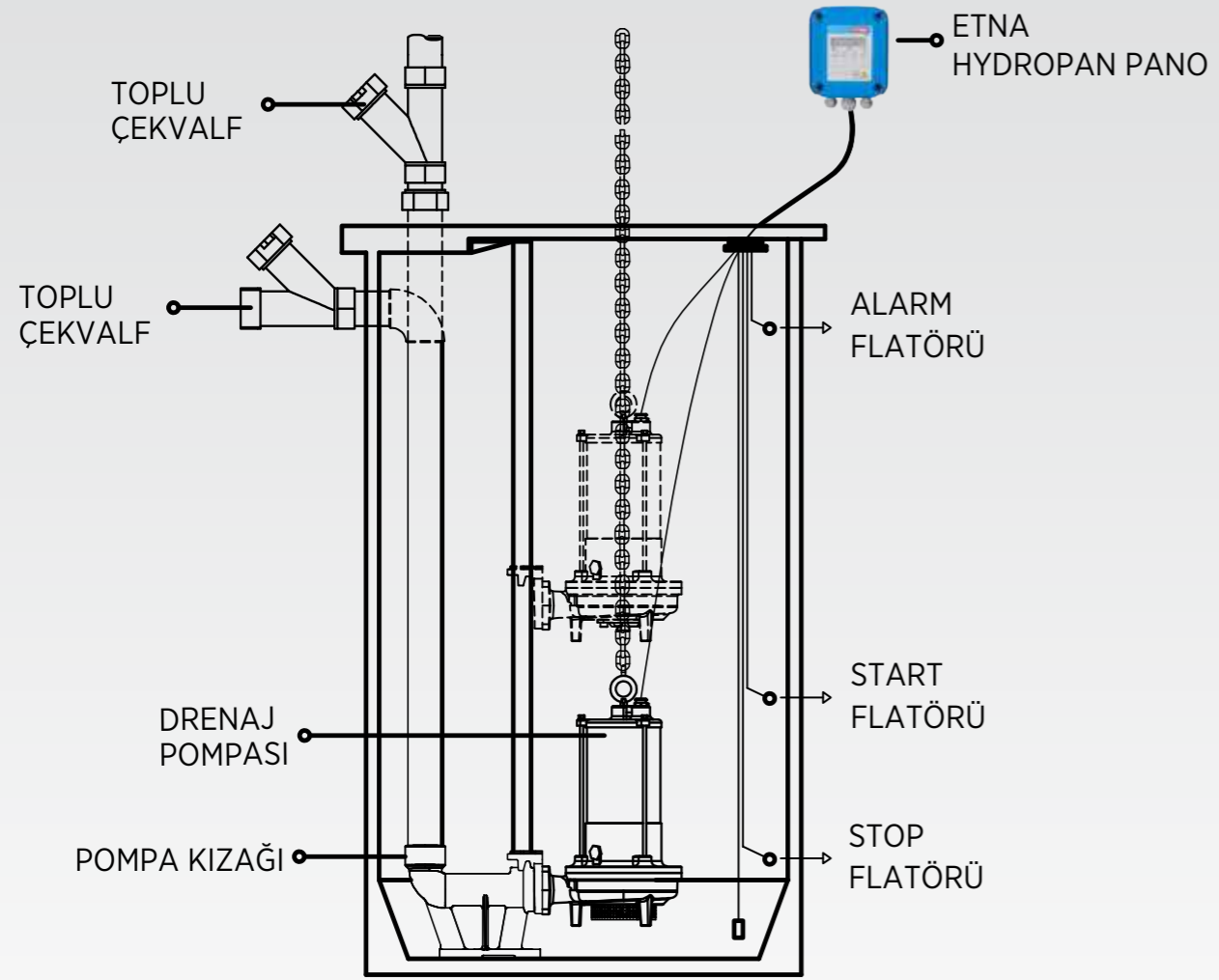
Kızaklı Sabit Tesisat (Servis ve Bakım İçin Kolay Çıkarılabilir Pompa)
